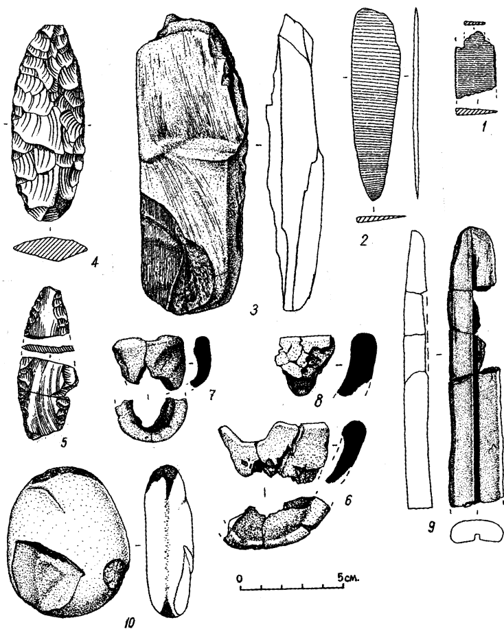
Рис. 11. Курья 1, 2 – ножи бронзовые, 4, 5 – ножи кремневые, 3 – абразивный камень, точило, 6–8 – обломки тиглей, 9 – глиняная форма, 10 – отбойник, камень.
